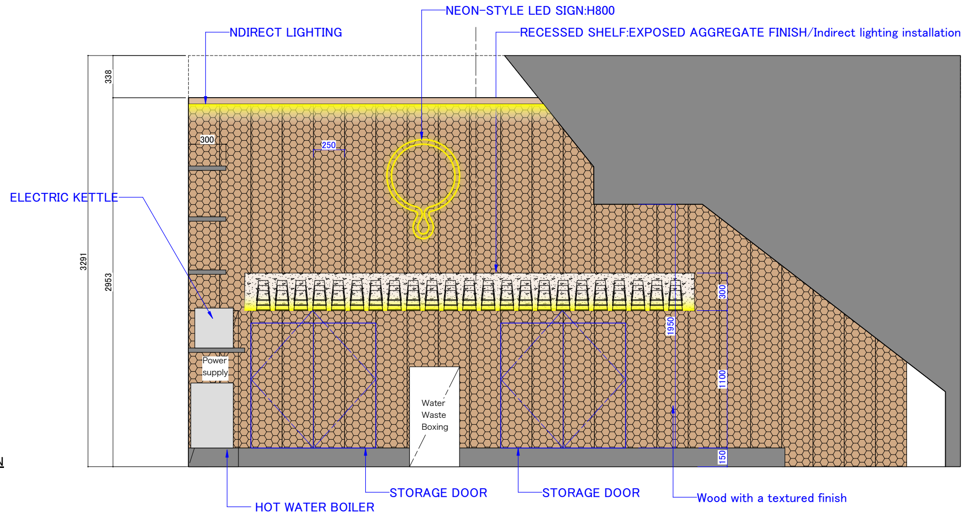
B ELEVATION
