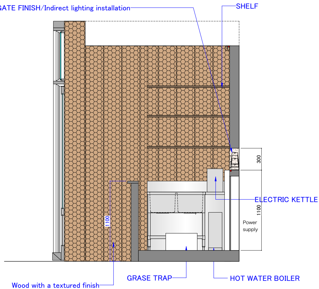
E ELEVATION
